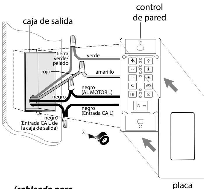
(cableado para el control de pared)
