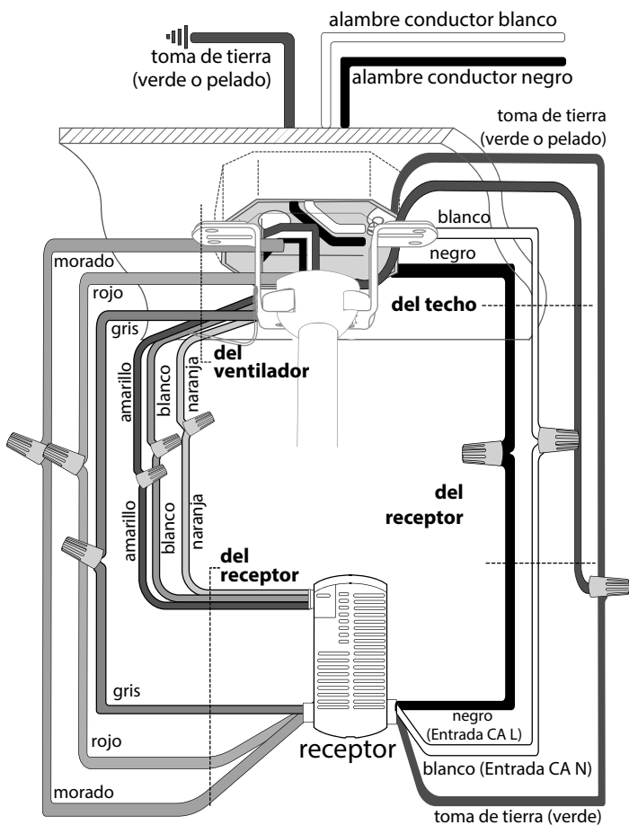
(cableado para el receptor)
